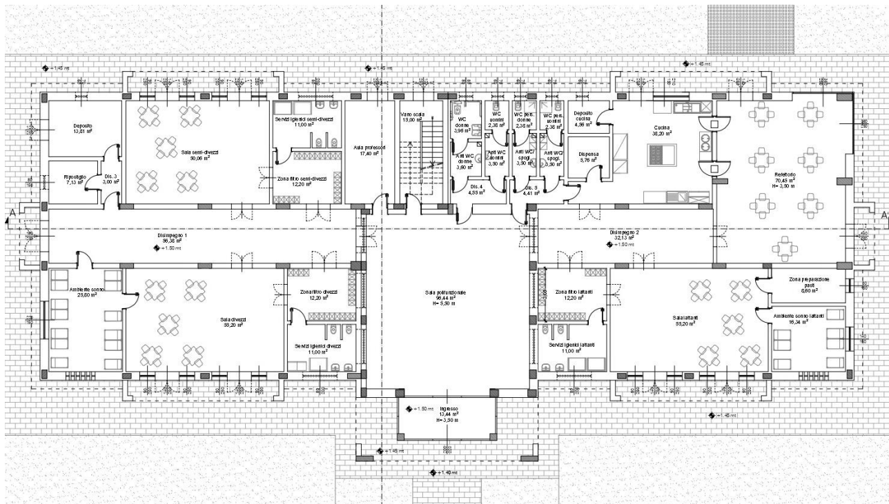
Planimetria del nuovo asilo di Calimera
